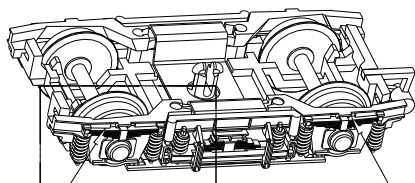
Federpakete – ausschwenkbar bei Kurvenfahrt nach Anschlag am Wagenboden.
