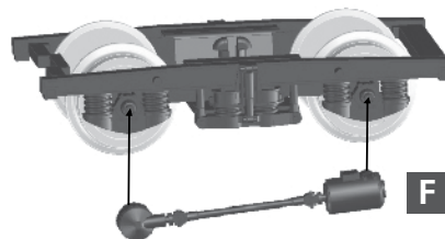
Drehgestell vollst. m. Kardanlichtmaschine 290938 Drehgestell vollst. o. Kardanlichtmaschine 290581
